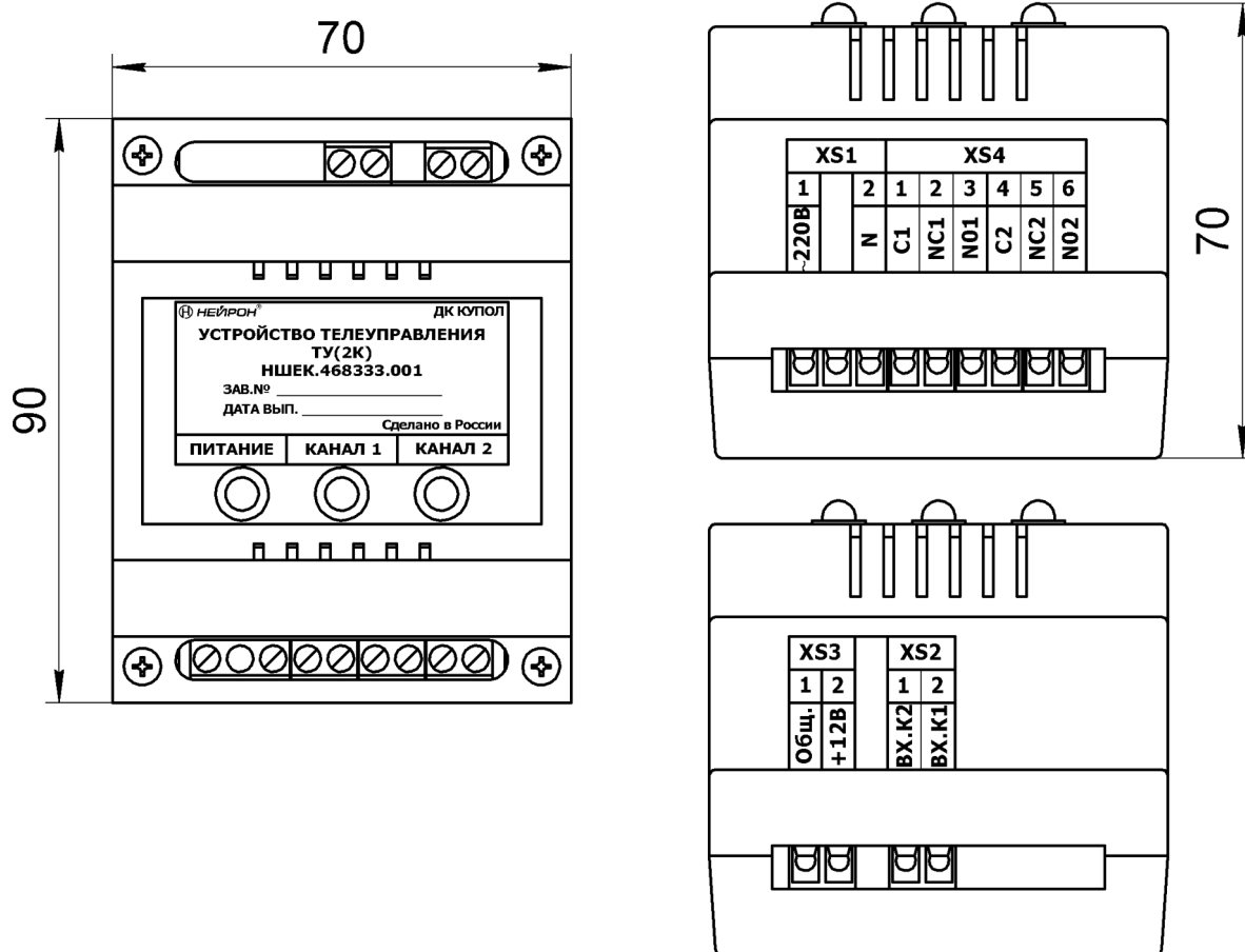
Рис.1 Внешний вид Устройства телеуправления ТУ(2К) НШЕК.468333.001
